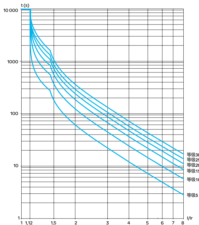
冷态脱扣曲线
