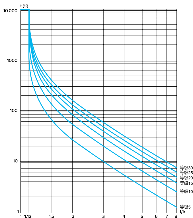
热态脱扣曲线
