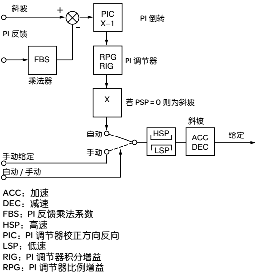
PI 调节器
